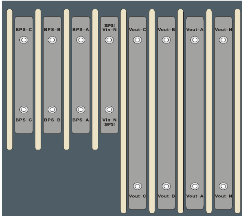
300kVA By-Pass girişı, çıkış bağlantısı için bakır çubuk
