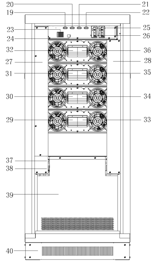
90kVA Arkadan Görünüm (kapaksız terminal bloğu)
